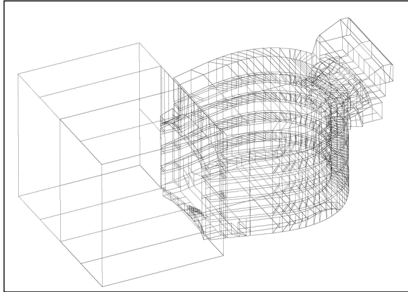
Figura 14 – Modelo geométrico tridimensional del Teatro Principal (AutoCAD)
