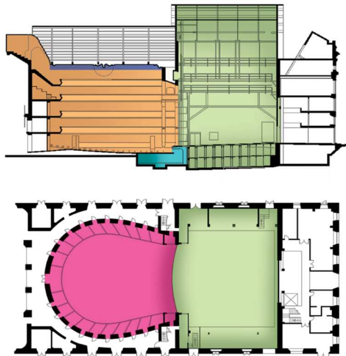
Figuras 3 y 4 - Rasgos morfológicos de la tipología teatral a la italiana señalados en la planimetría del Teatro Principal de Valencia (Barba y Giménez, 2011a, pp. 36-37)
