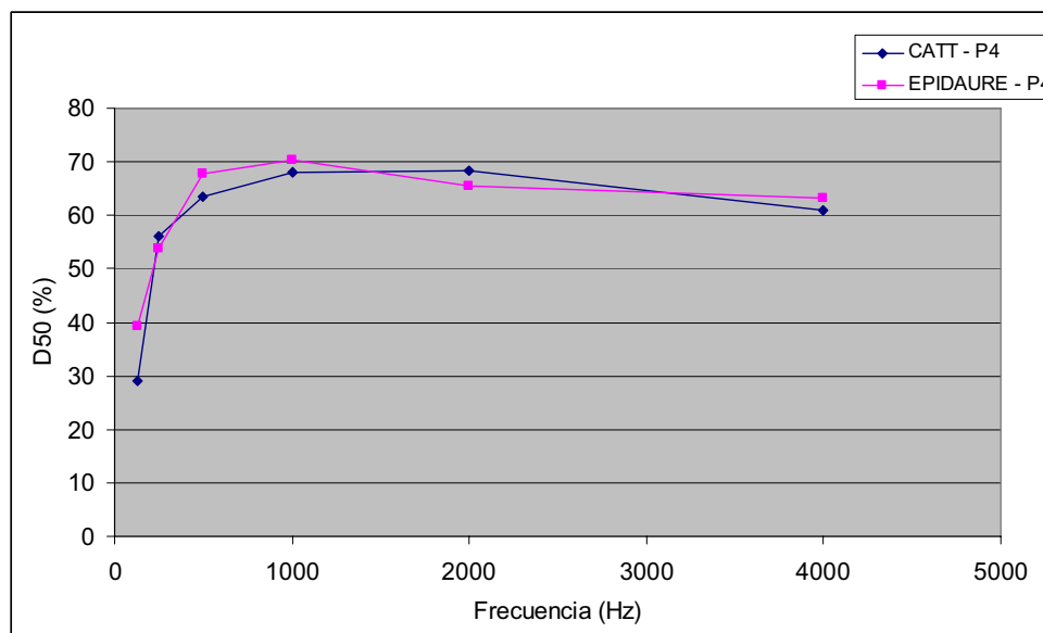
Figura 7 – Gráfico de D50 calculados con CATT y EPIDAURE en la posición P4
