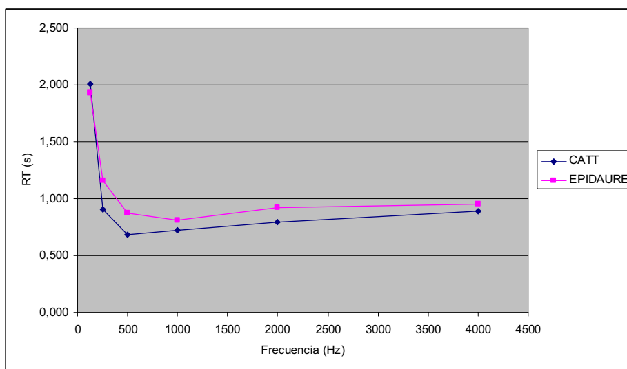
Figura 6 – Gráfico de los RT calculados con CATT y EPIDAURE
