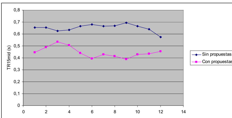
Figura 4 – Gráfico de los RT15mid con propuestas y sin propuestas
